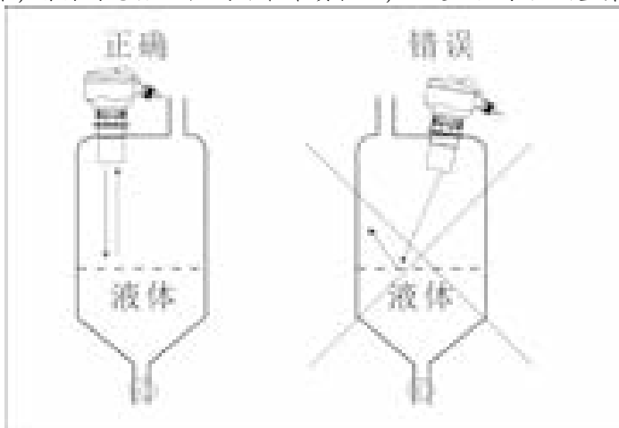
传感器探头应垂直于介质表面
