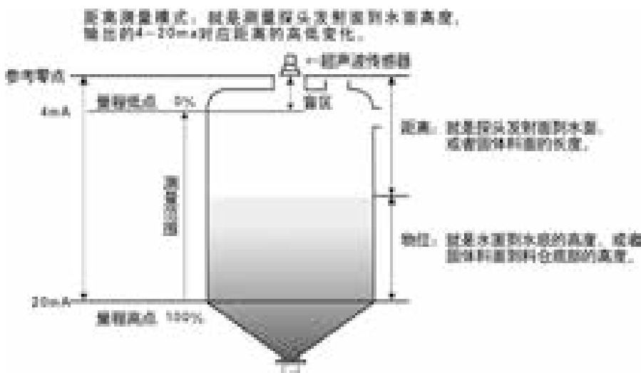
附图 1.1 距离测量示意图
