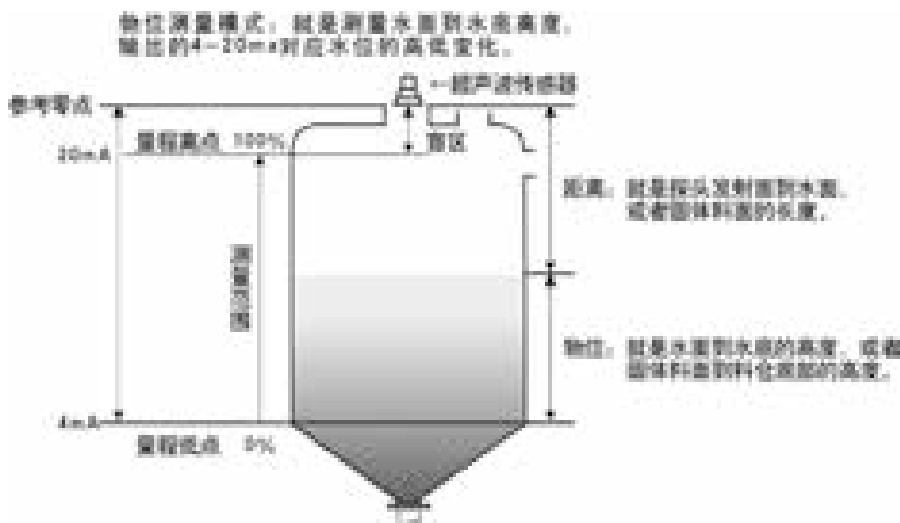
附图 1.2 物位测量示意图
