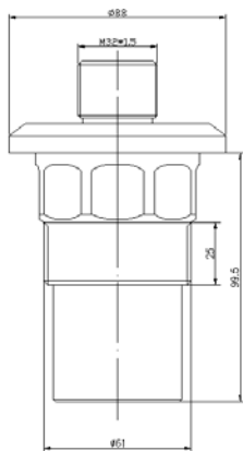
G2 寸螺纹
