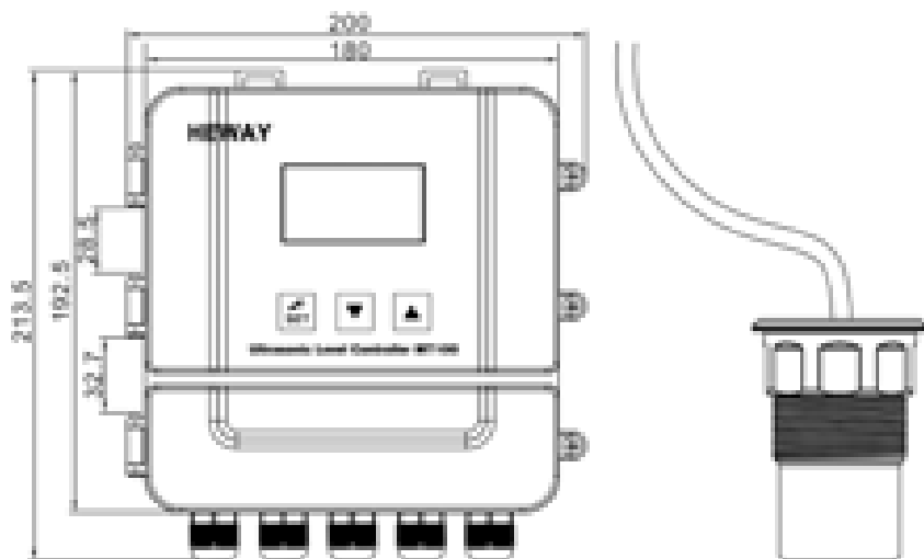
结构图
