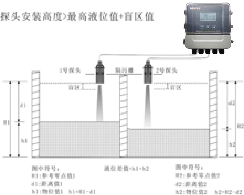
附图 1.3 液位差计和双通道液位计测量示意图
